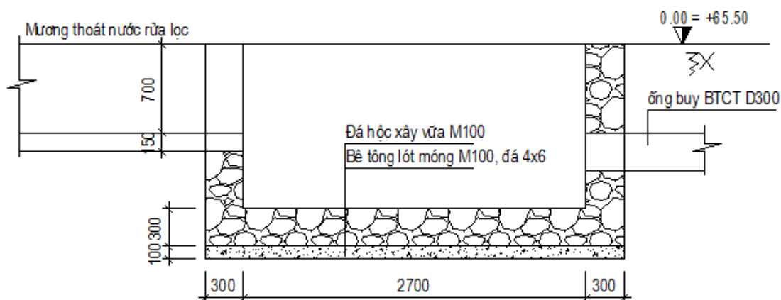
Hình 3.2. Mặt cắt hệ thống xử lý nước thải
