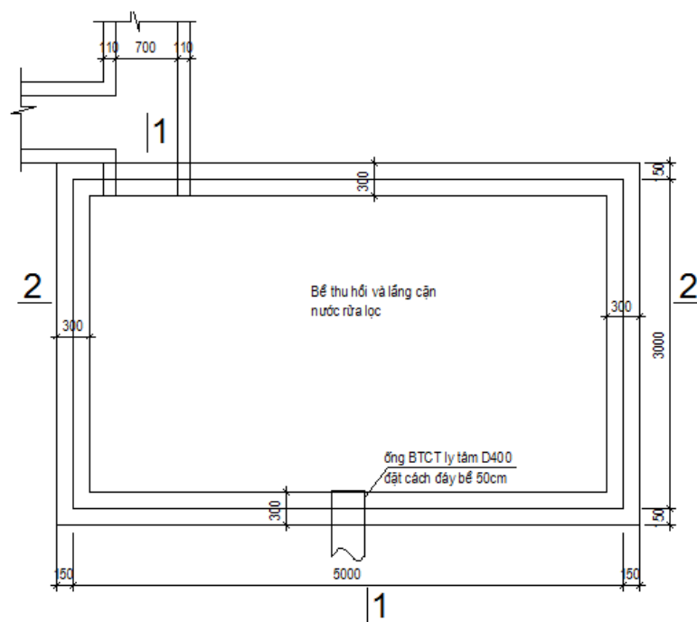
Hình 3.1. Mặt bằng hệ thống xử lý nước thải
