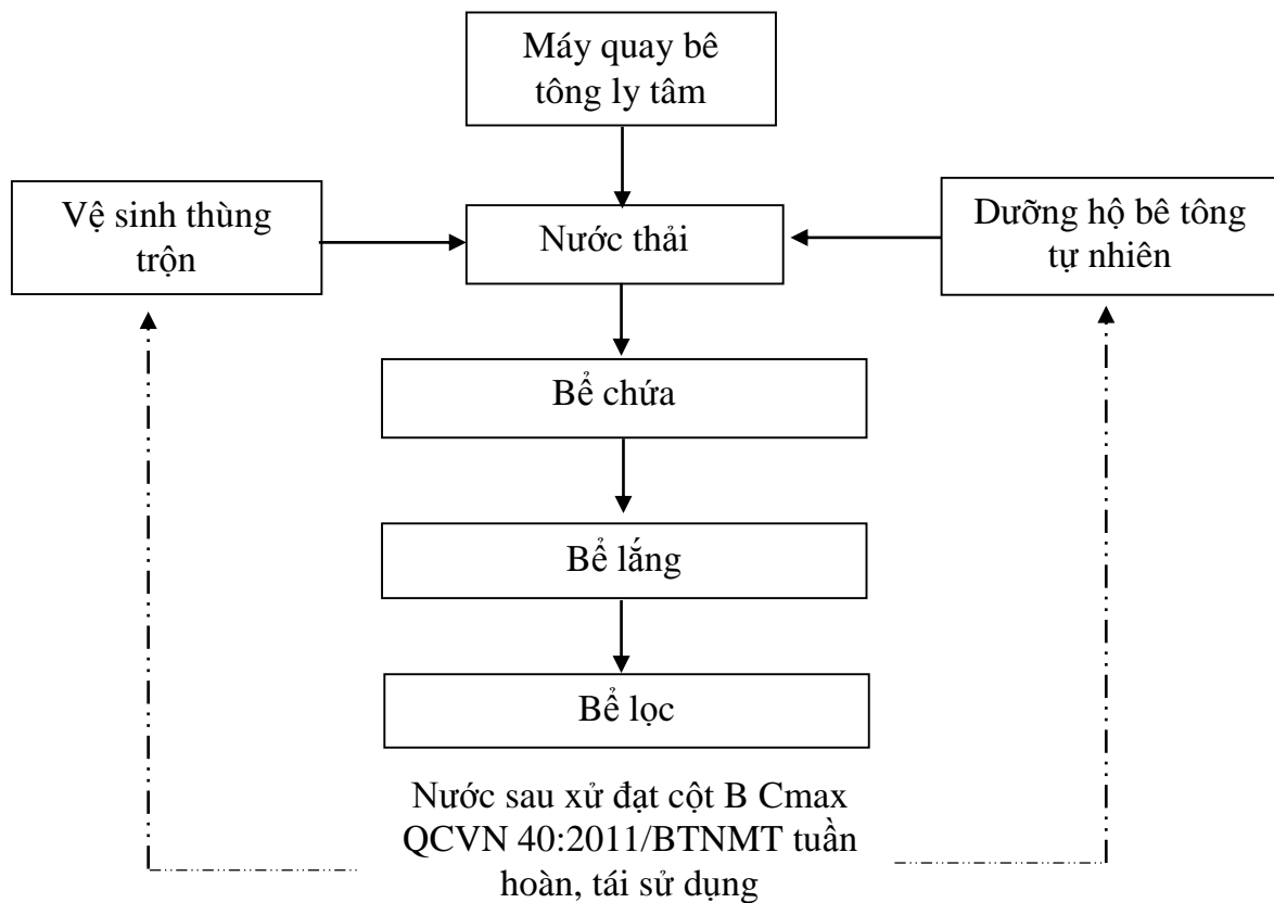
Hình 12. Quy trình xử lý nước thải sản xuất của Cơ sở
