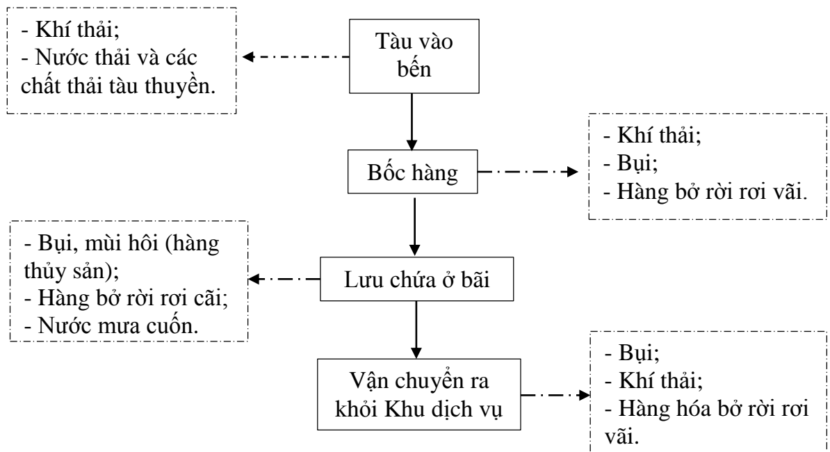
Hình 5. Quy trình hoạt động bốc hàng tại bãi chứa hàng hoá
