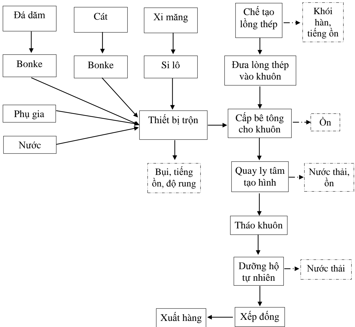
Hình 3. Quy trình sản xuất cấu kiện bê tông
