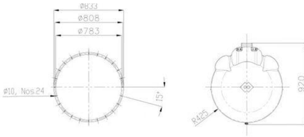
Hình 14. Cấu tạo thiết bị lọc bụi silo xi măng
