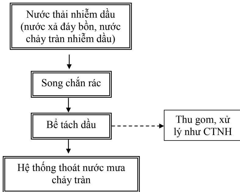
Hình 20. Sơ đồ xử lý nước thải nhiễm dầu
