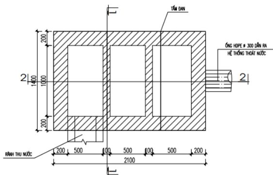
MẶT BẰNG BỂ LẮNG DẦU. TL : 1-25
