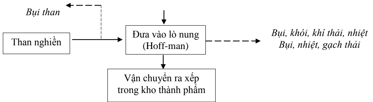
Hình 3. Sơ đồ quy trình sản xuất gạch Tuynel
