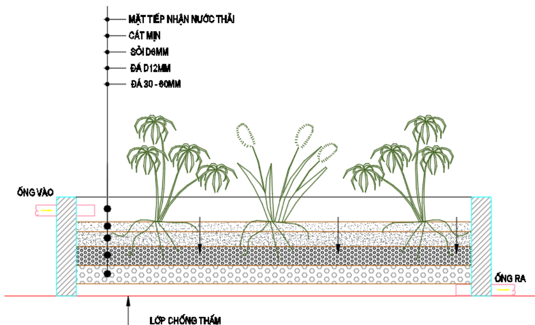
Hình 19. Cấu tạo bể lọc ngầm trồng cây
