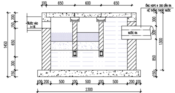
MẶT CẮT 2-2. TL : 1-25
